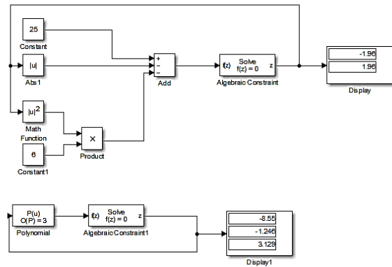
Рис. 2. Модель устройства для решения уравнений, созданная в Simulink
