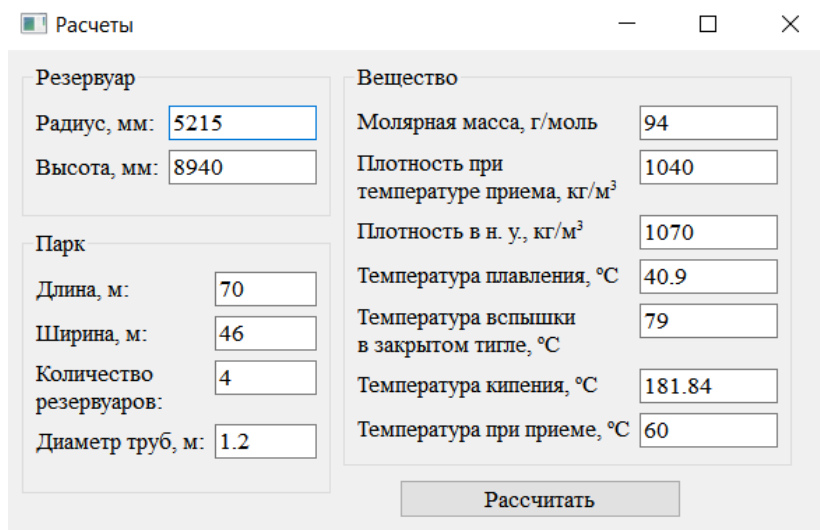
Рис. 3. Окно «Расчеты»
