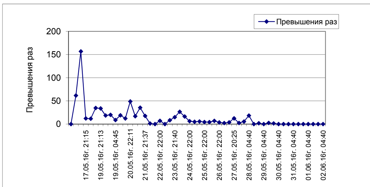
Рис. 2. Динамика концентраций сероводорода в атмосферном воздухе в ночное время
