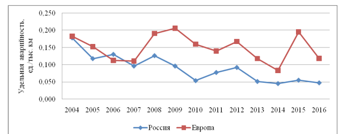
Рисунок 2 — Динамика удельной аварийности на магистральных газопроводах России (БД Ростехнадзор) и стран Европы (БД CONCAWE) [5, 9]
