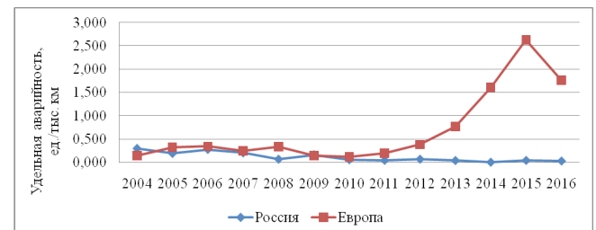
Рисунок 1 — Динамика удельной аварийности на магистральных нефтепроводах России (БД Ростехнадзор) и стран Европы (БД CONCAWE) [6, 9].
