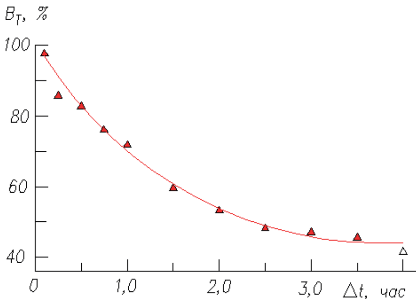
Рисунок 6. Зависимость выхода по току от продолжительности электролиза: i_k = 15 \text{ A/м}^2
