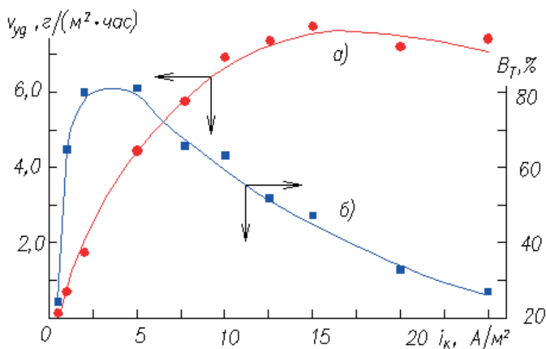
Рисунок 2. Зависимость скорости формирования Mg(OH)_2 и выхода по току от плотности катодного тока в режиме гальваностатирования (продолжительность электролиза — 3 часа)
