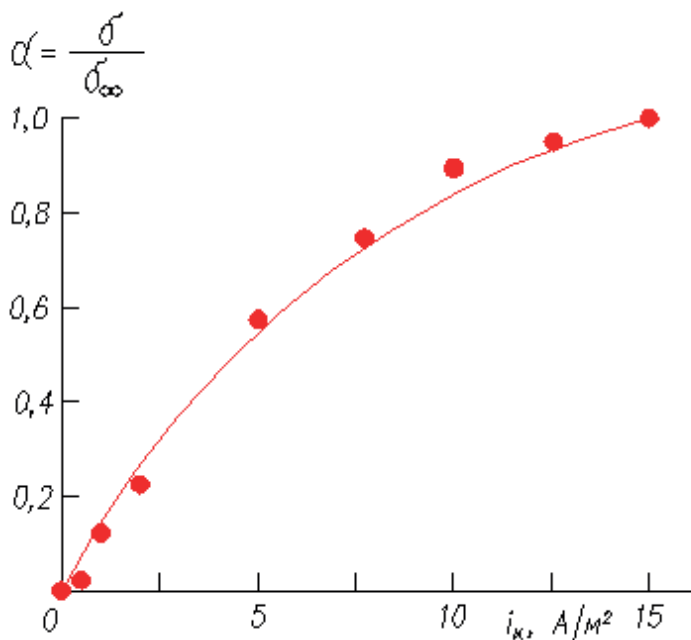
Рисунок 4. Зависимость степени превращения от плотности катодного тока
