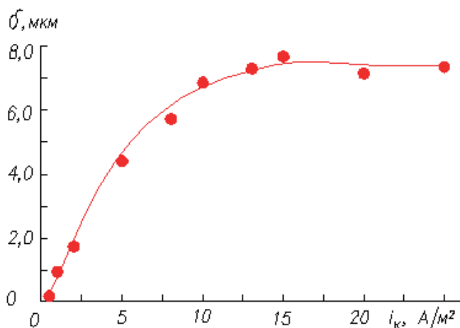
Рисунок 3. Зависимость толщины покрытия от плотности катодного тока в режиме гальваностатирования (продолжительность электролиза — 3 часа)
