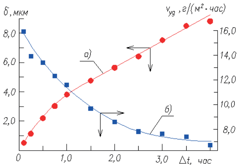
Рисунок 5. Зависимость толщины покрытия (а) и удельной скорости формирования слоя Mg(OH)_2 (б) от продолжительности электролиза: i_k = 15 \text{ A/м}^2 .
