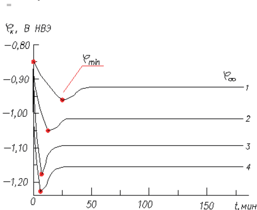
Рисунок 1. Изменение во времени катодных потенциалов при различных плотностях катодного тока: i_k = 2,0 (1); 5,0 (2); 15,0 (3) и 25,0 \text{ А/м}^2 (4).
