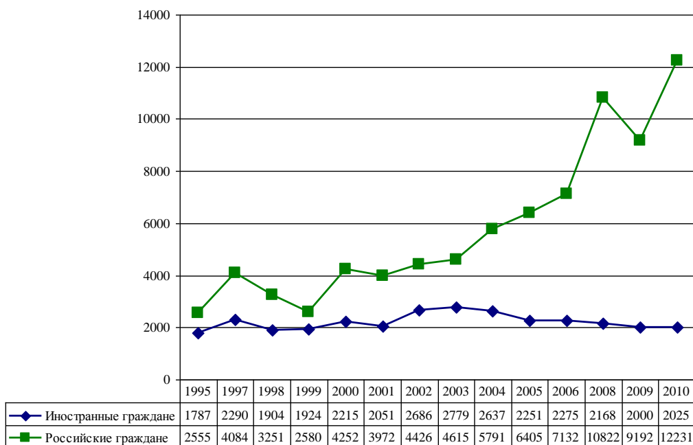
Рис. 1. Динамика численности международных туристских обменов России
