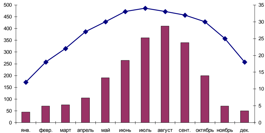
Рис. 4. Изменение уровня влажности и температуры на севере Вьетнама
