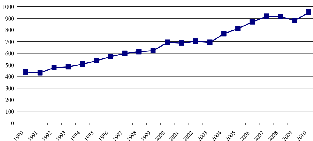
Рис. 2. Динамика международных туристских потоков за период 1990 – 2010 гг.
