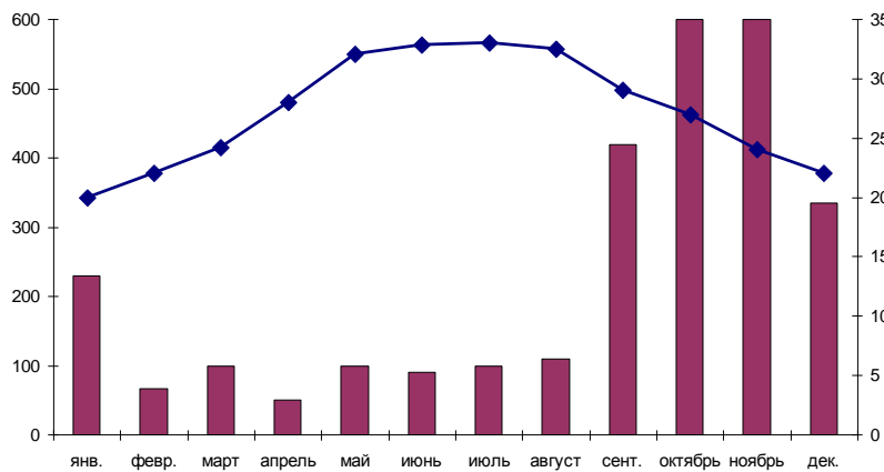
Рис. 5. Изменение уровня влажности и температуры в центральном Вьетнаме
