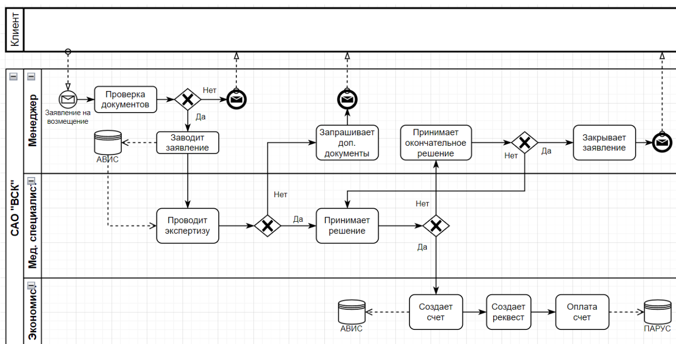
Рис. 2. Модель бизнес-процесса
