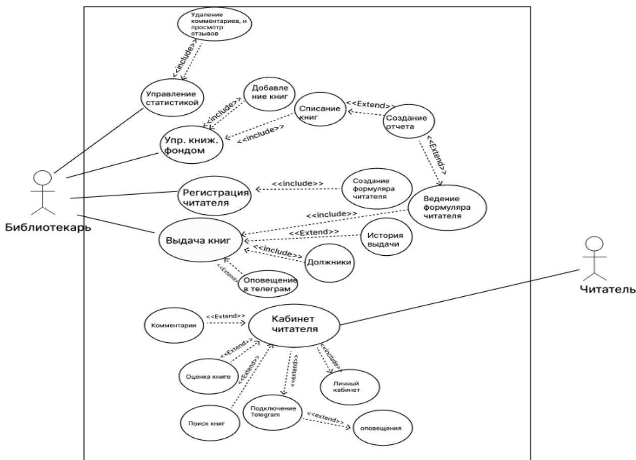
Рис. 1. Диаграмма вариантов информационной системы
