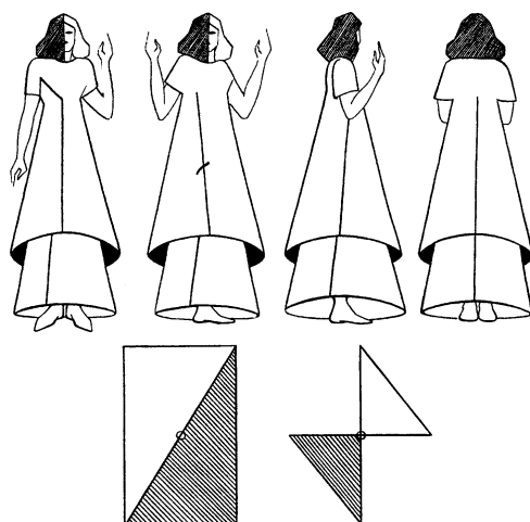
Рис. 15. Поворотная симметрия
