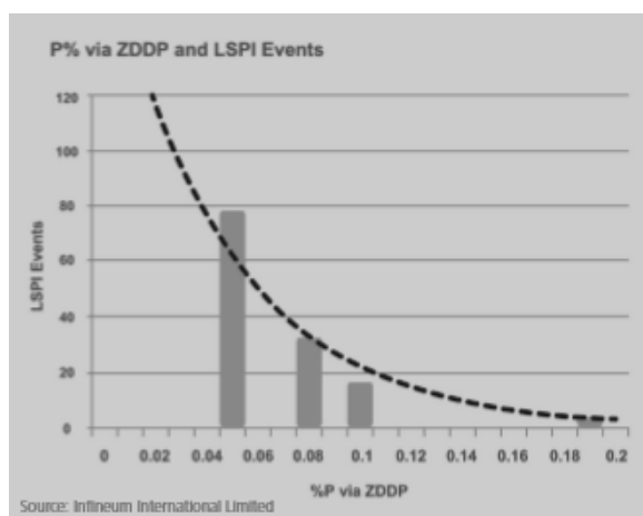
Рис. 2. Влияние диалкилдитиофосфата цинка на вероятность ПВСЦ
