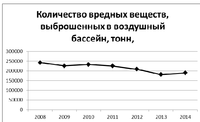
Рис. 3. Количество вредных веществ, выброшенных в воздушный бассейн
