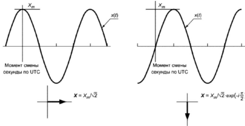
Рис. 1. Представление синхронизированного вектора [4]:
