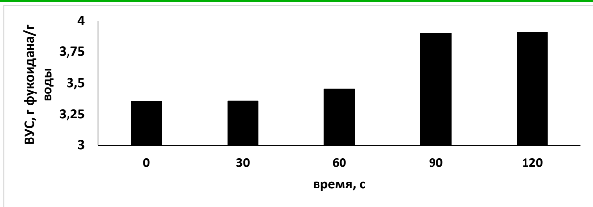
Рис. 1. Влияние времени обработки микроволновым излучением на ВУС фукоидана
