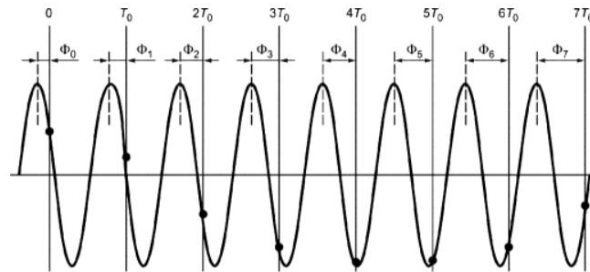
Рис. 3. Изменение фазового угла синхронизированного вектора
