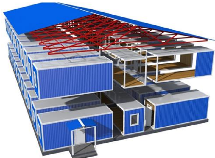
Рис. 4. Устройство блочно-модульного сооружения
