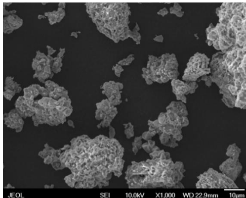
Рис. 3. РЭМ-изображение частиц гидросиликата кальция после обжига при температуре 1100°C.
