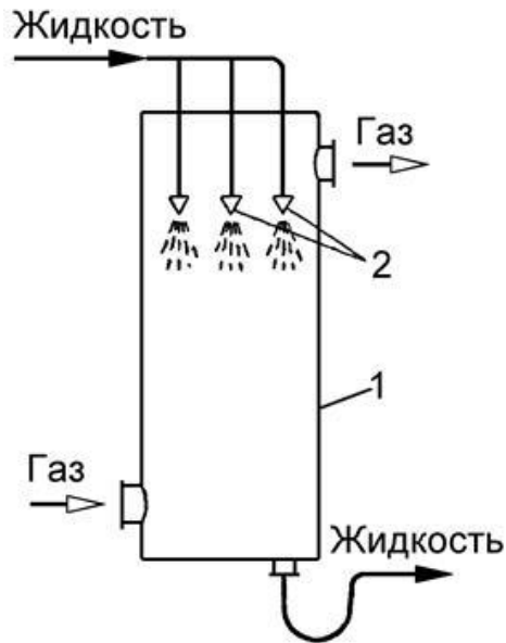
Рис. 1. Абсорбер
