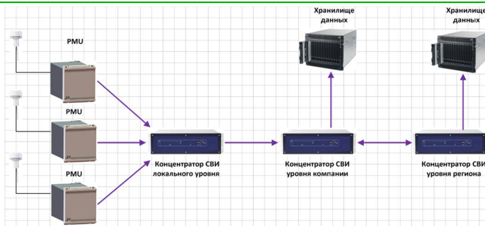
Рис. 5. Типовая архитектура системы синхронизированных векторных измерений [10]
