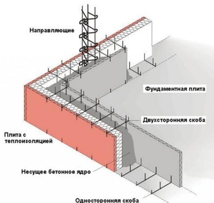
Рис. 1. Устройство несъемной опалубки
