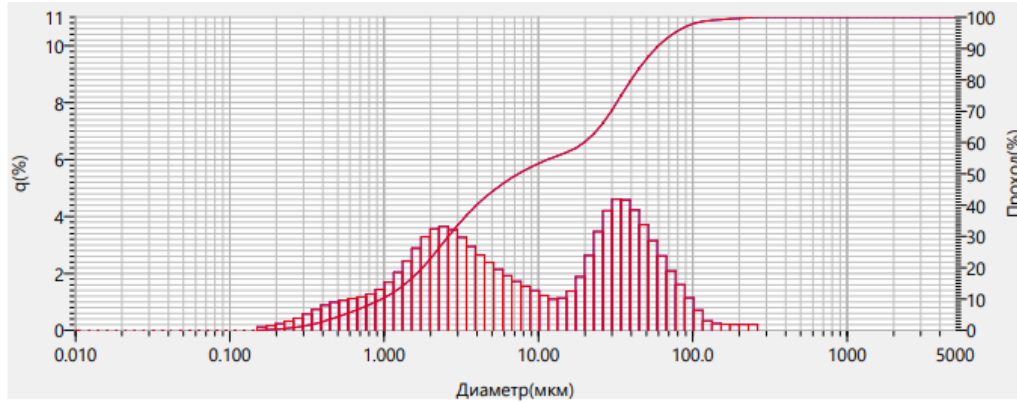
Рис. 2. Дисперсный состав шихты.
