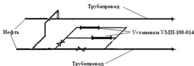
Рис. 2. Схема монтажа установок для обработки нефти электромагнитным полем.
